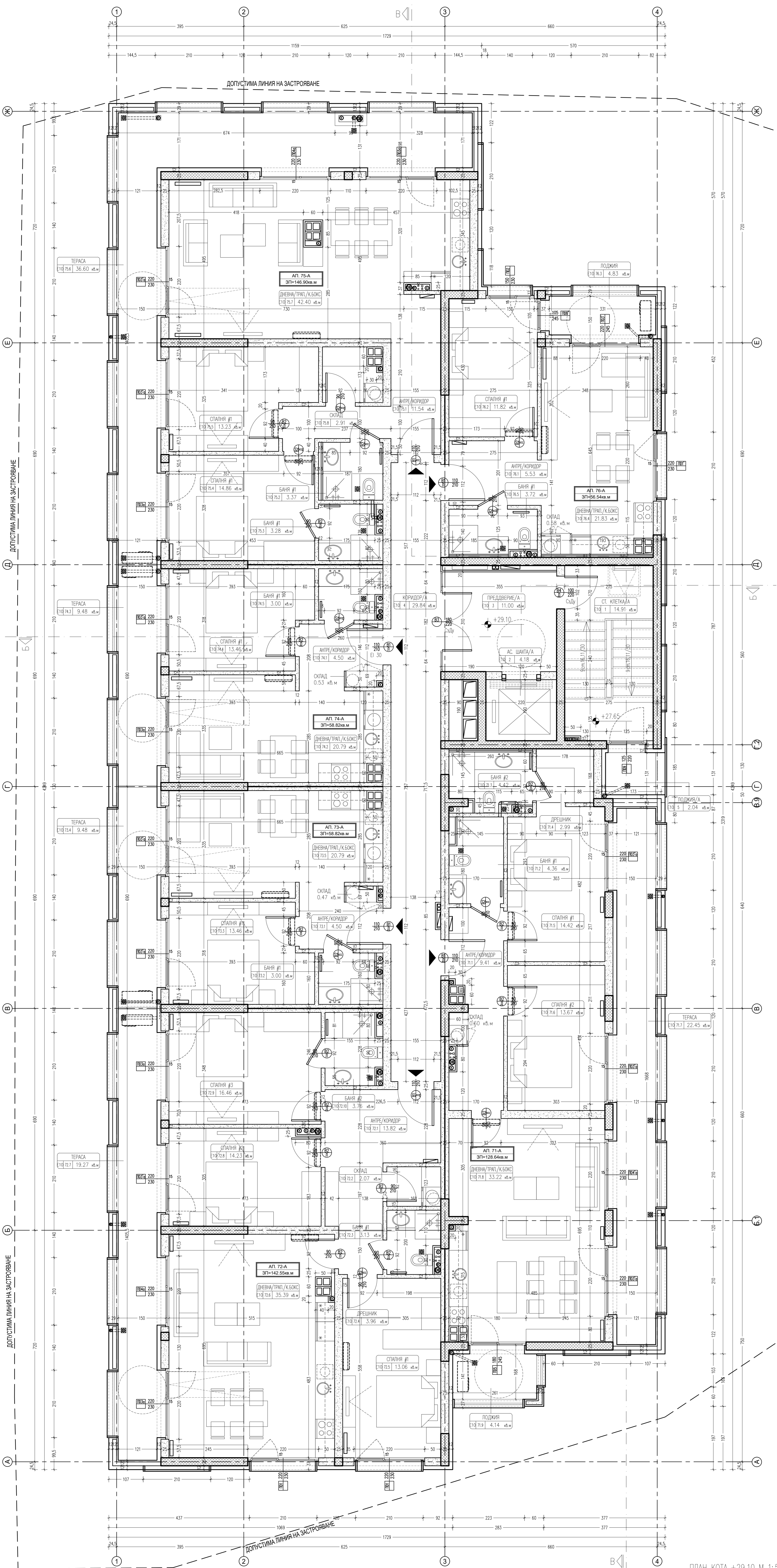
ПЛАН КОТА +29.10 М 1:50
